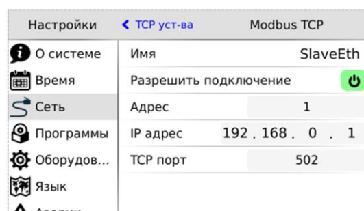
Рис. 72 – Настройка Modbus-TCP slave
