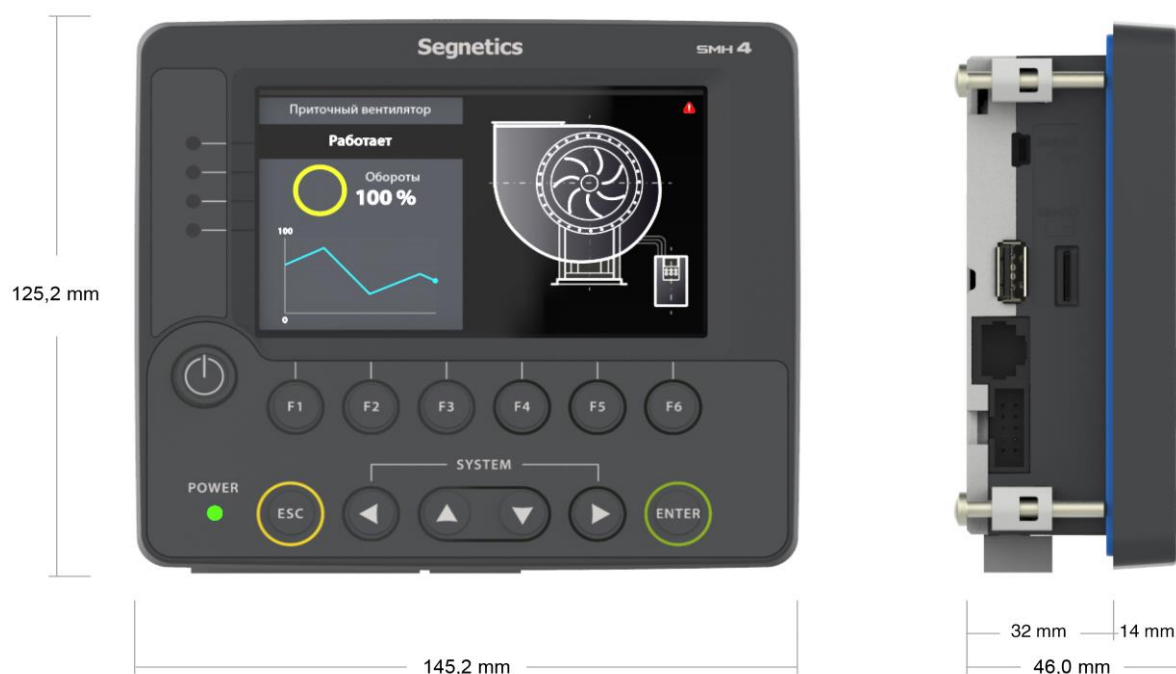
Рис. 5 – Габаритные размеры контроллера без модуля MC
