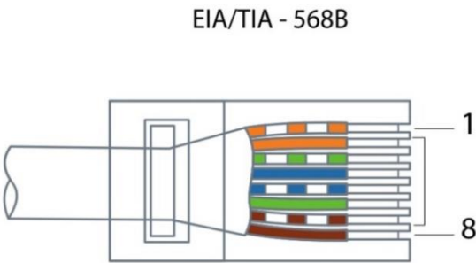
Рис. 54 – Нумерация проводников в кабельном разъёме
