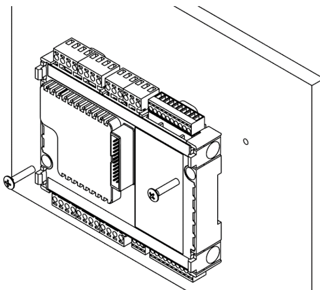
Рис. 20 – Фиксация модуля MC к панели винтами
