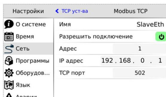
Рис. 69 – Экран настроек Slave
