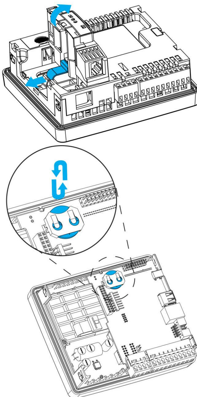
Рис. 16 – Порядок замены литиевой батареи
