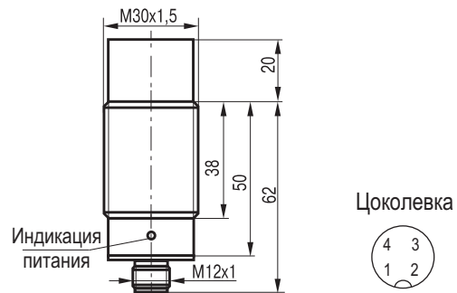
Габаритный чертеж
