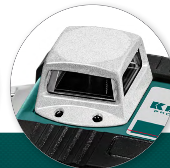
Металлический кожух лазерных блоков
