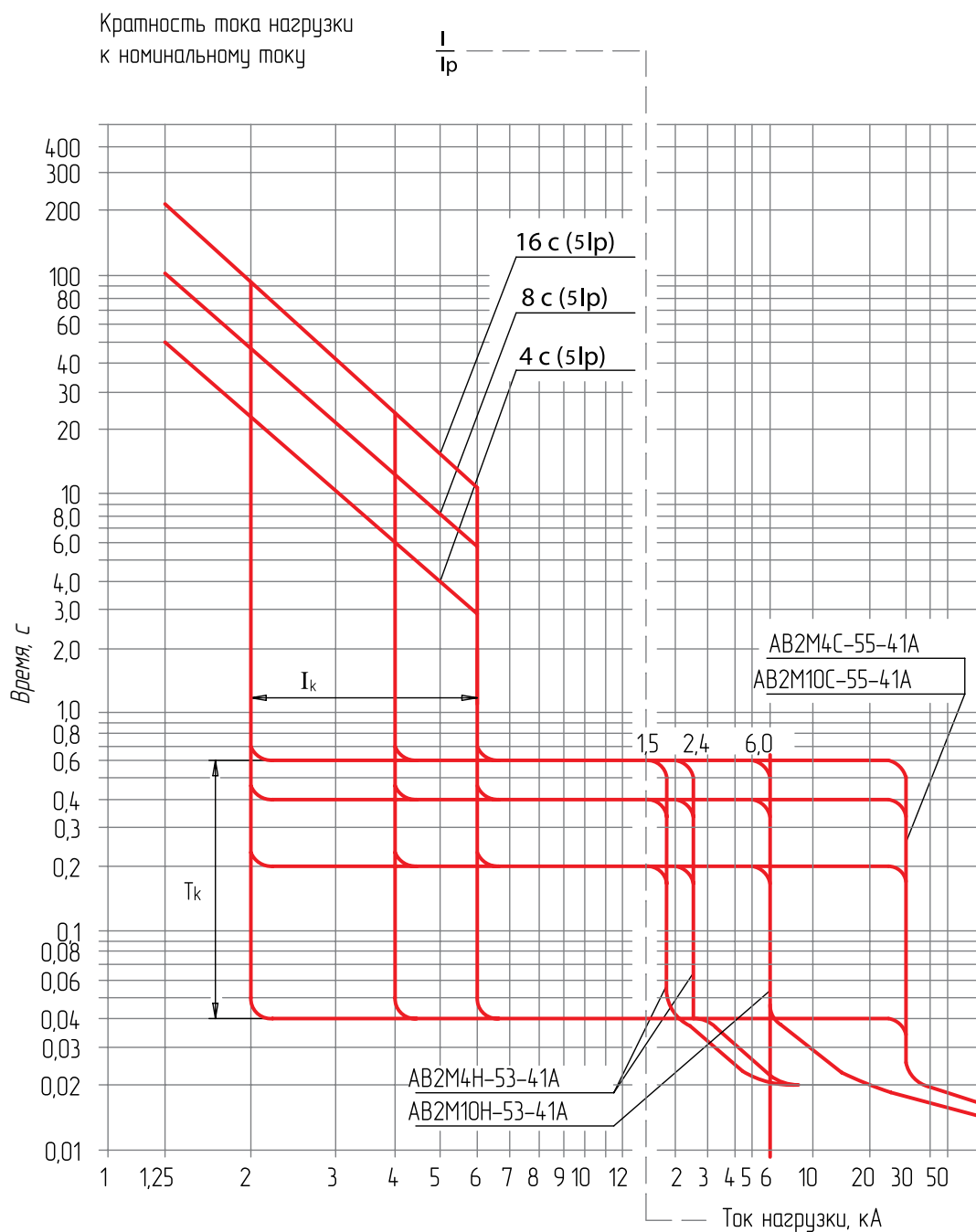
Рисунок В.2. Времятоковые характеристики выключателей постоянного тока
