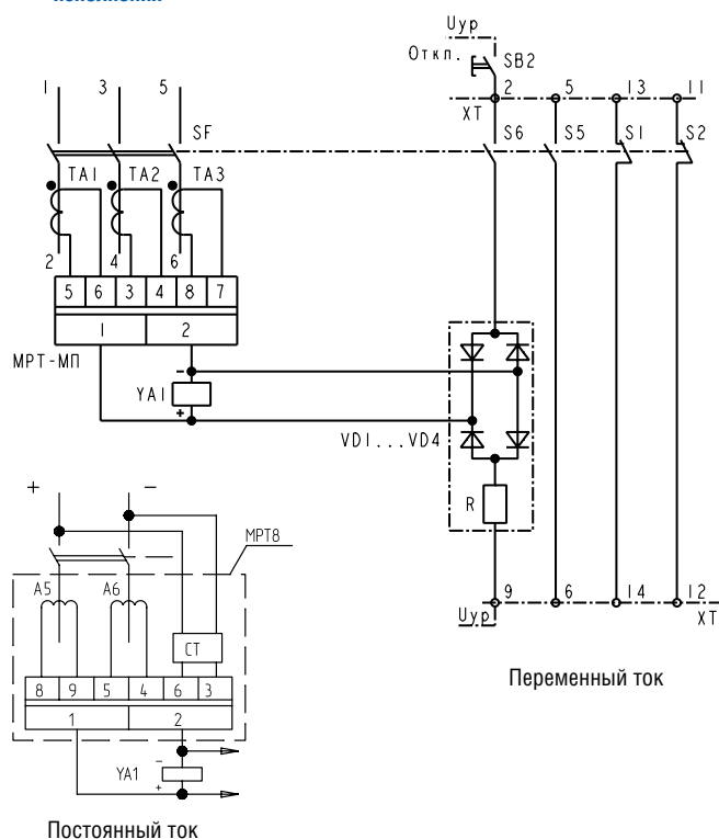
Рисунок Б.1. Схема электрическая принципиальная выключателей с ручным приводом и независимым расцепителем стационарного исполнения
