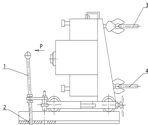
Рисунок 13. Выкатывание выключателя выдвижного исполнения
