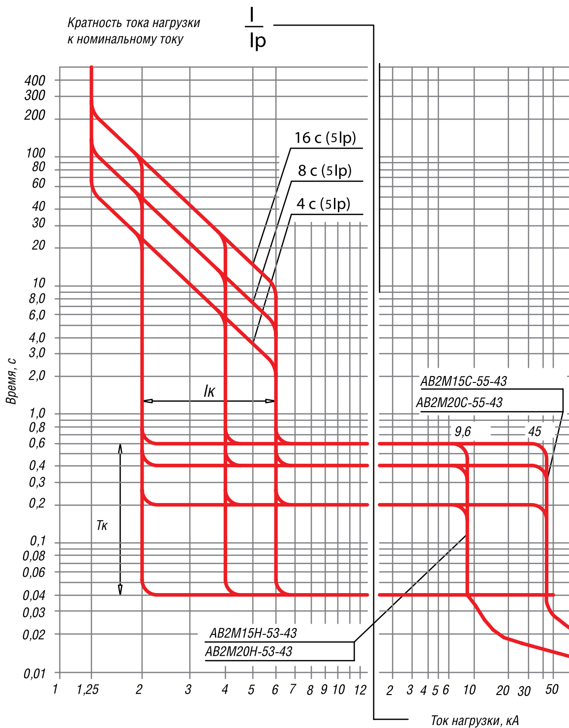
Рисунок В.4. Временные характеристики выключателей постоянного тока
