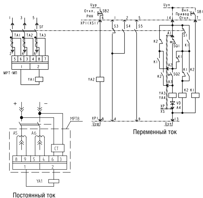
Рисунок Б.8. Схема электрическая принципиальная выключателей с электроприводом и нулевым расцепителем выдвижного исполнения
