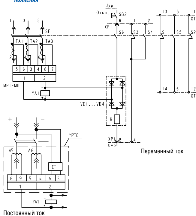
Рисунок Б.4. Схема электрическая принципиальная выключателей с ручным приводом и независимым расцепителем выдвижного исполнения
