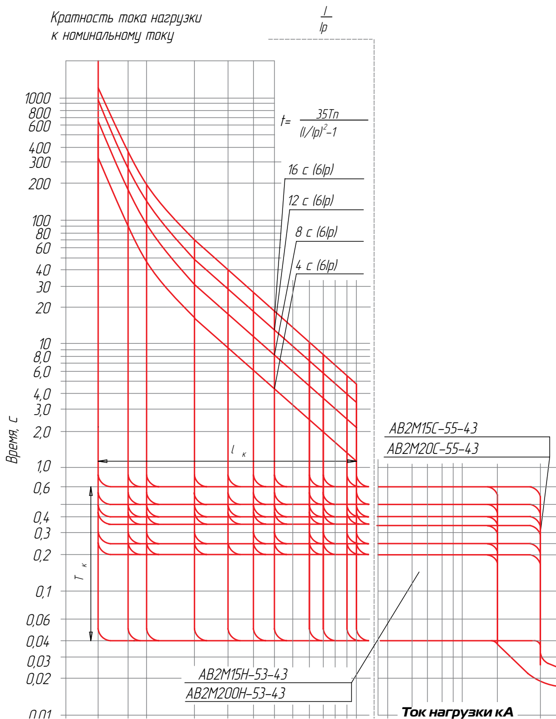
Рисунок В.3. Временные характеристики выключателей переменного тока с блоком МРТ4-МП (обратноквадратичная характеристика защиты от перегрузки)
