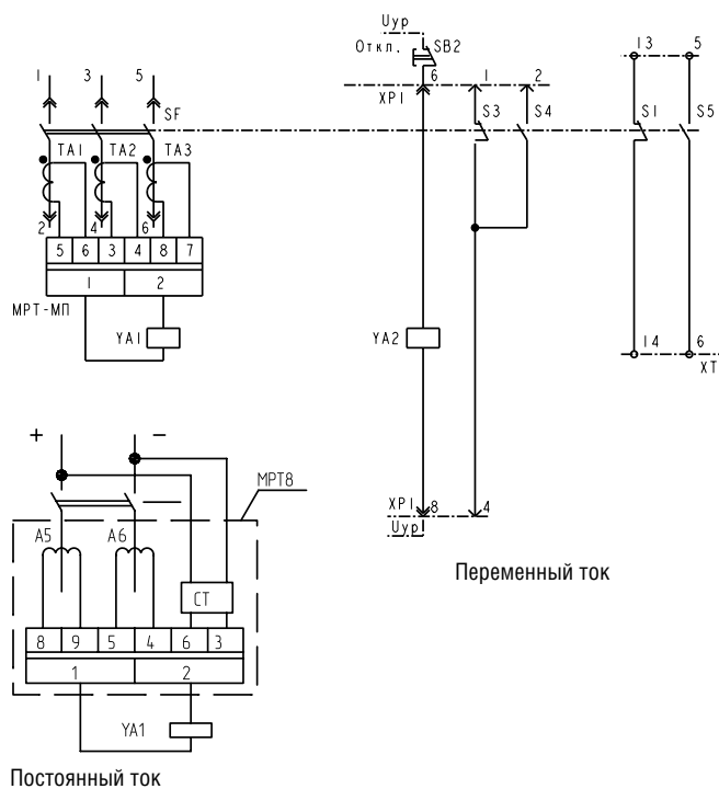
Рисунок Б.5. Схема электрическая принципиальная выключателей с электроприводом и независимым расцепителем стационарного исполнения
