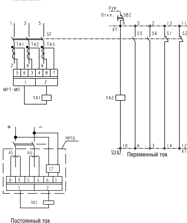
Рисунок Б.2. Схема электрическая принципиальная выключателей с ручным приводом и нулевым расцепителем стационарного исполнения
