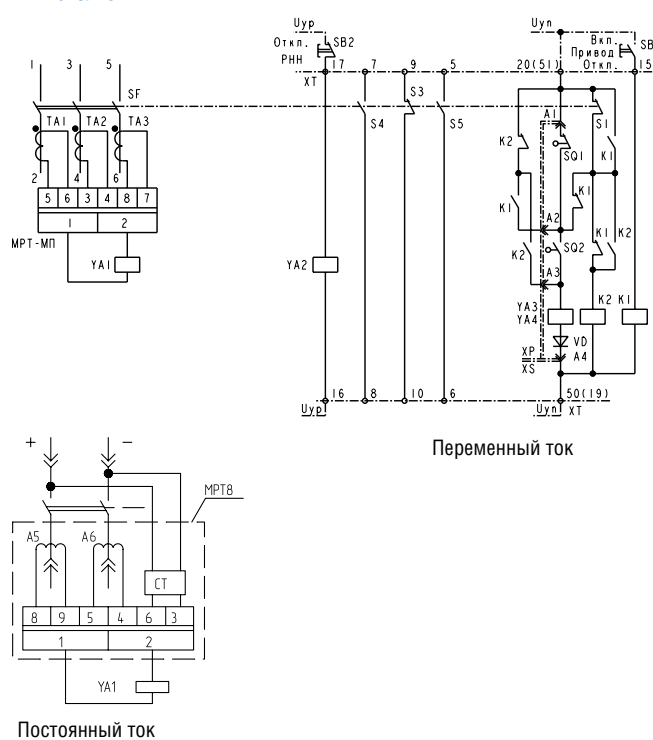
Рисунок Б.6. Схема электрическая принципиальная выключателей с электроприводом и нулевым расцепителем стационарного исполнения
