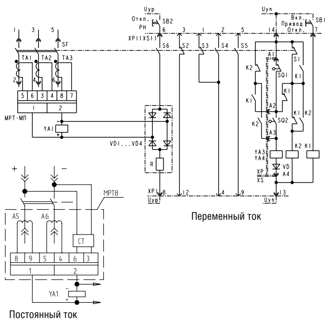
Рисунок Б.7. Схема электрическая принципиальная выключателей с электроприводом и независимым расцепителем выдвижного исполнения
