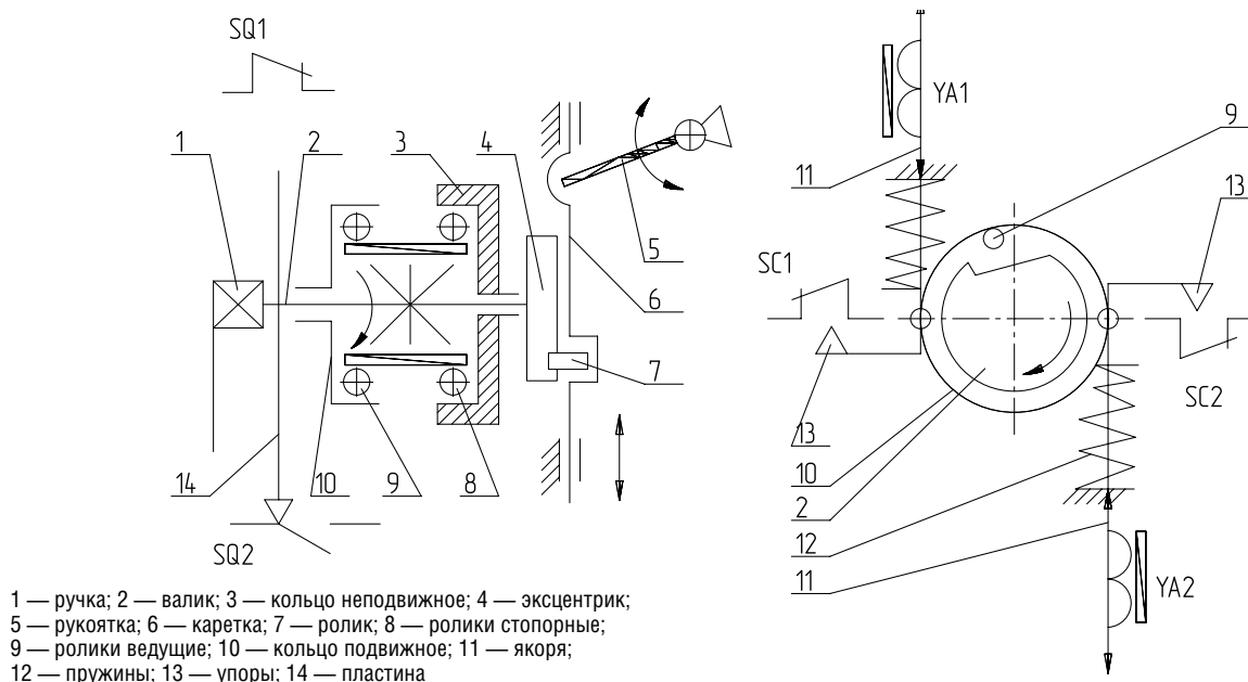
Рисунок 8. Схема привода кинематическая
