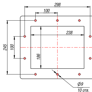
Выходной фланец
