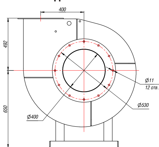
Выходной фланец
