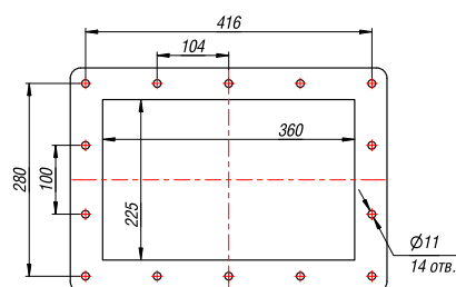
Выходной фланец
