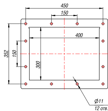
Выходной фланец
