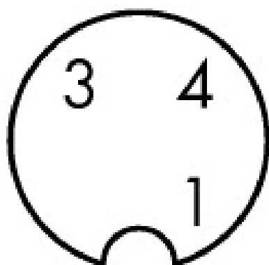
M12-Buchse
