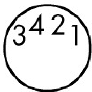
M8-Buchse
