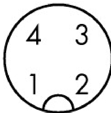
M12-Stecker
