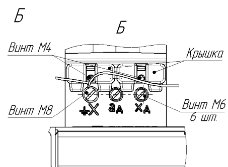
Рисунок А.3 Общий вид трехфазной группы 3хЗНОЛП
