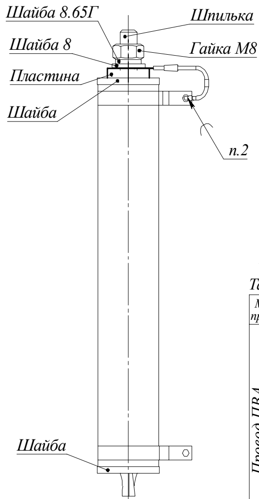
Рисунок Б.1 Установка резистора
