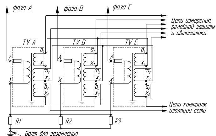
Рисунок А.4 Принципиальная электрическая схема трехфазной группы 3хЗНОЛП
