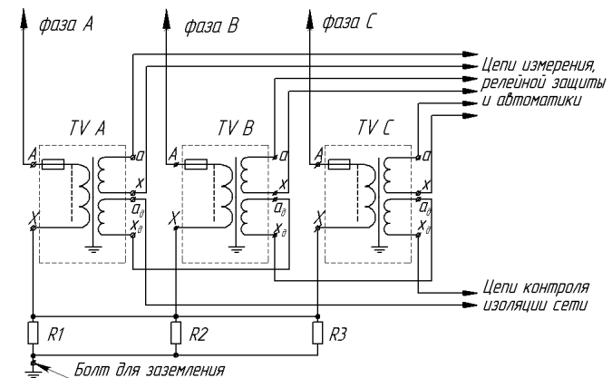
Рисунок А.2 Принципиальная электрическая схема трехфазной группы 3хЗНОЛП
