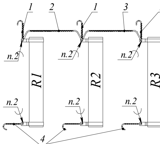
Рисунок Б.2 Монтажная схема соединения резисторов
