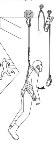
Рис. 3д. Перережьте строп
