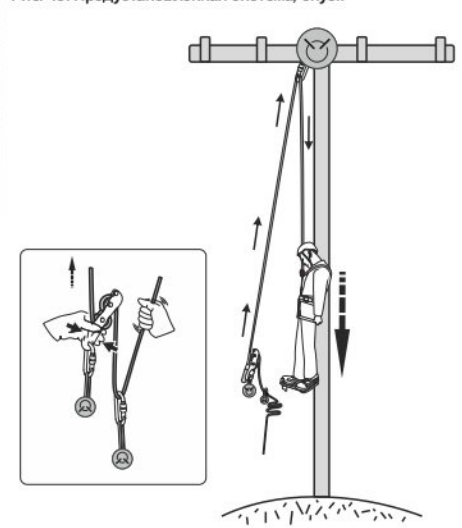
Рис. 4б. Предустановленная система, спуск
