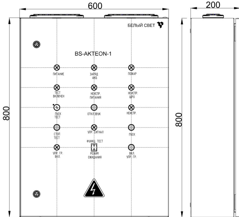
Рис. №1 Габаритный чертёж.
