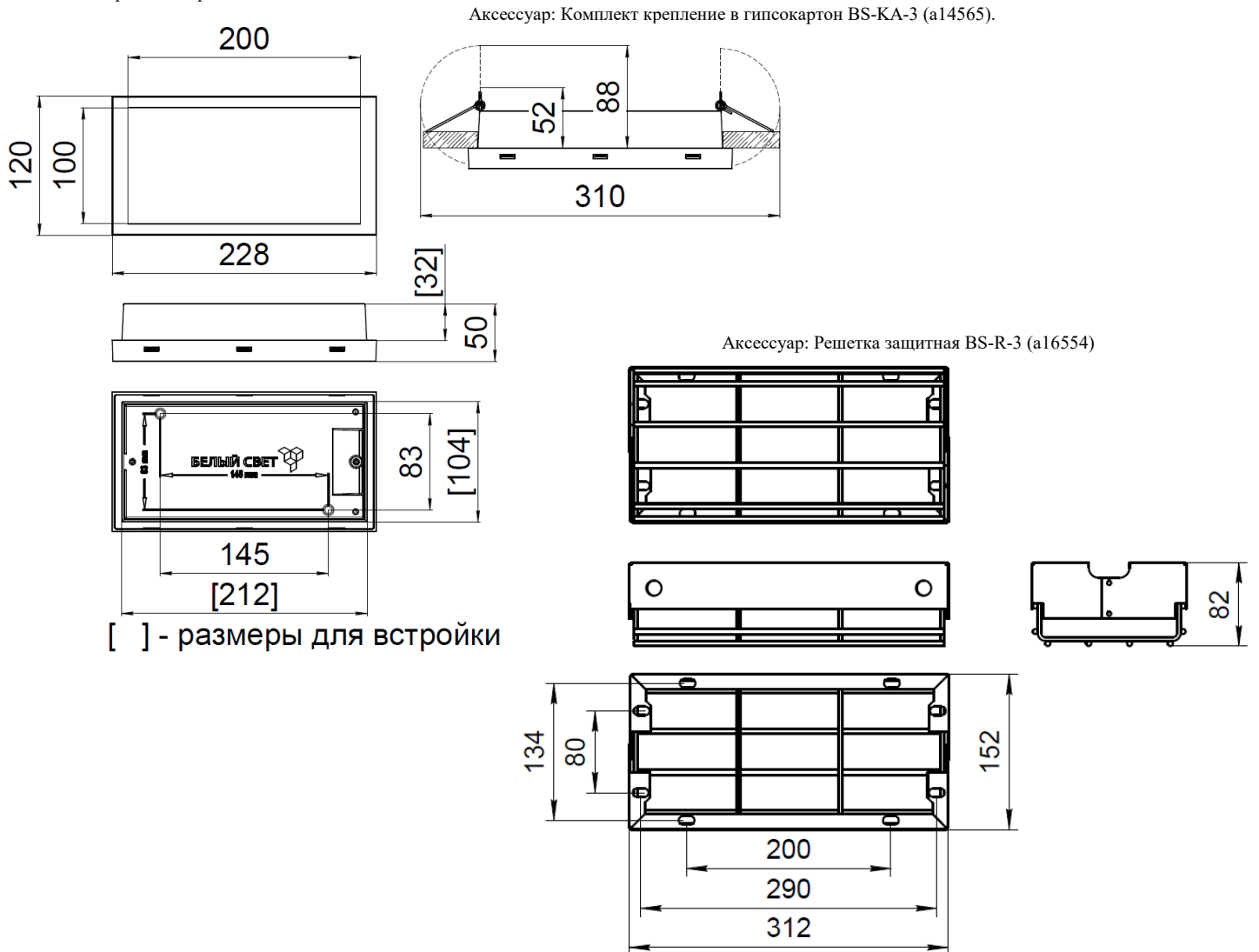
Рис. №2 Габаритный чертёж.
