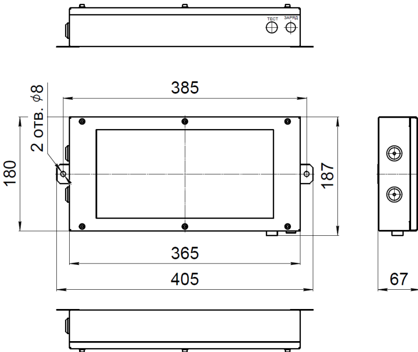
Рис. №3 Габаритный чертёж.
