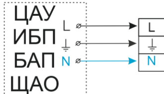
Рис. №2 Схема подключения BS-CANRON-10-S2 (-60C)
