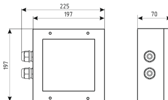
Рис. №2 Габаритный чертёж.
