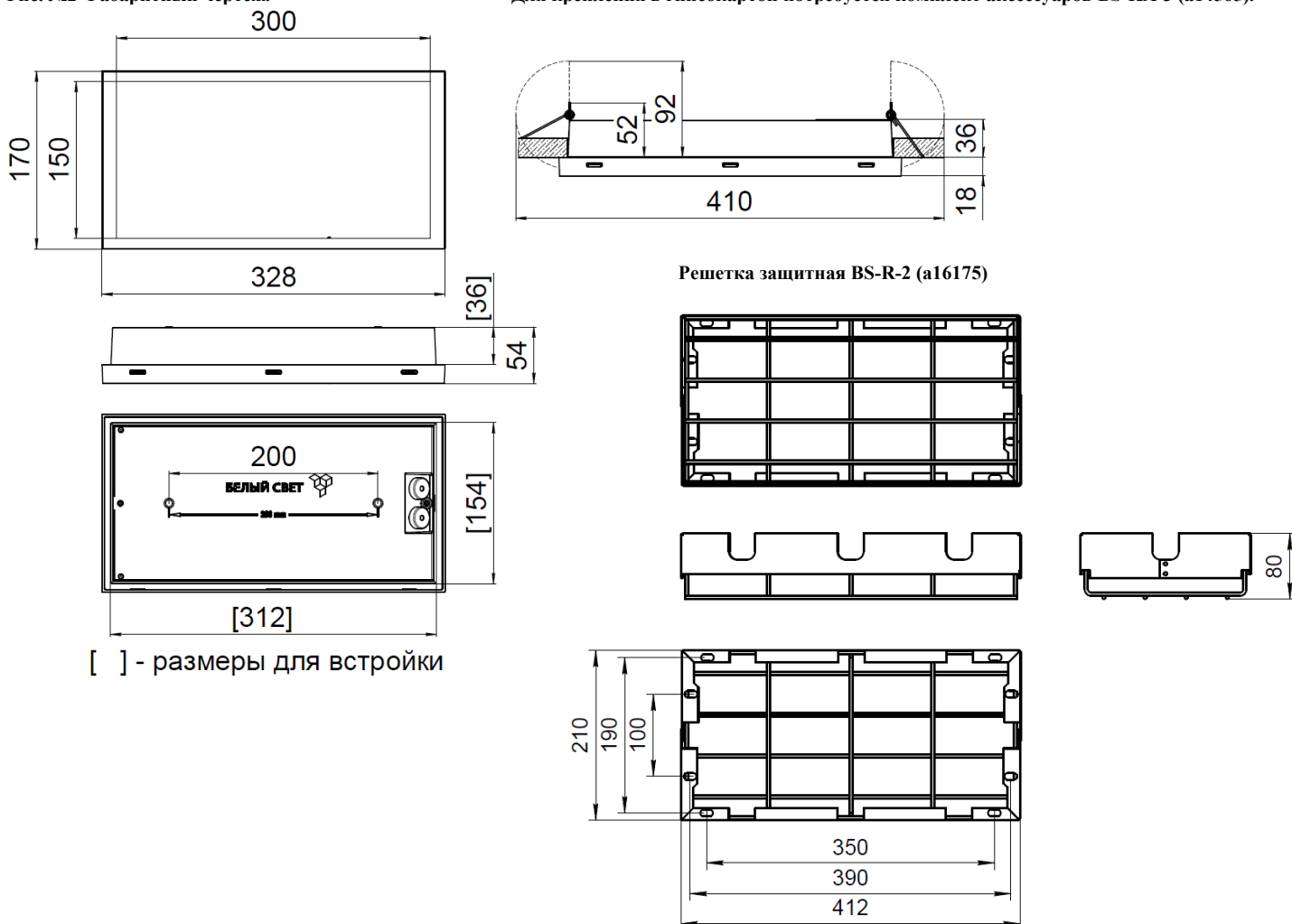
Рис. №2 Габаритный чертёж.
