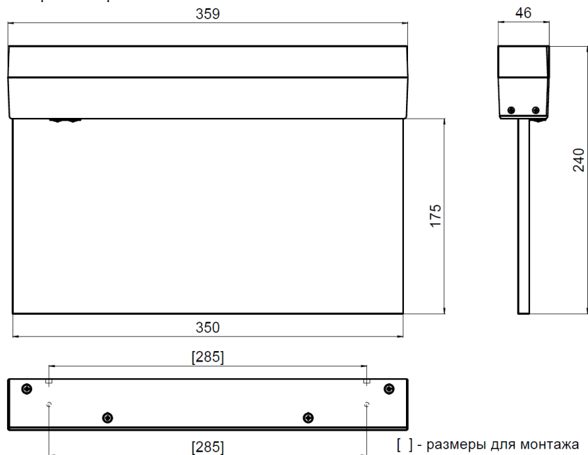
Рис. №2 Габаритный чертёж.
