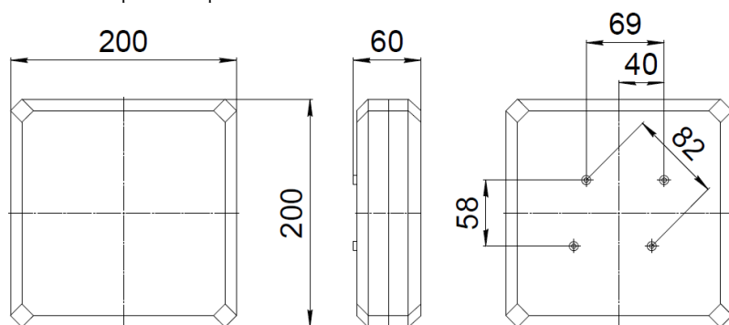
Рис. №2 Габаритный чертёж.
