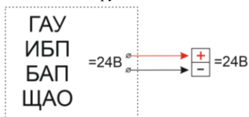
Рис. №1 Схема подключения к групповой цепи питания.
