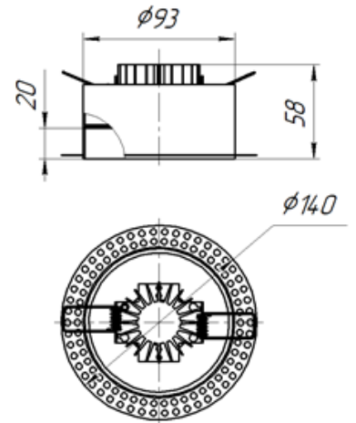
Рис. №3 Аксессуары Стакан потолочный BS-SP-1
