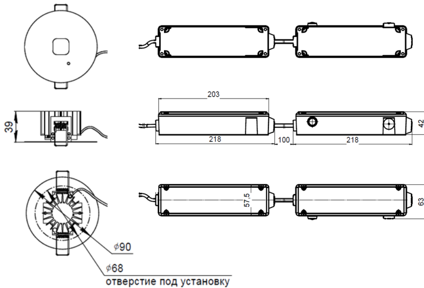
Рис. №2 Габаритный чертёж.
