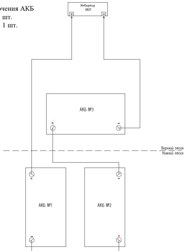
Рис. №2 Схема подключения аккумуляторных батарей.
