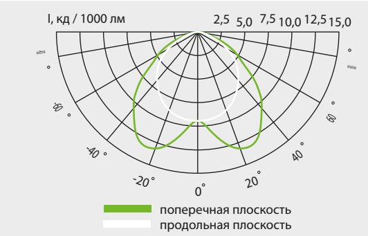
Светотехнические характеристики
