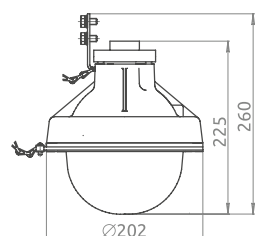
КОРОТКИЙ КОЛПАК
