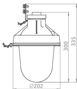
ДЛИННЫЙ КОЛПАК
