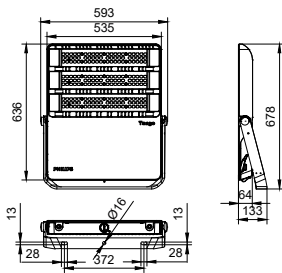
BVP384 LED614/NW 490W 220-240V AMB GM
