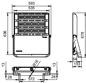
BVP384 LED528/840 490W 220-240V AMB GM
