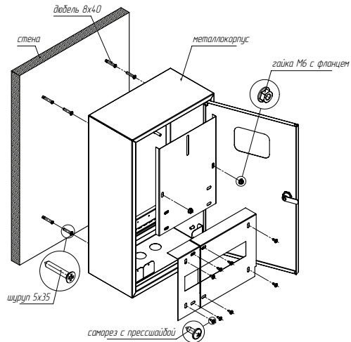
Рис. 1 - Схема монтажа
