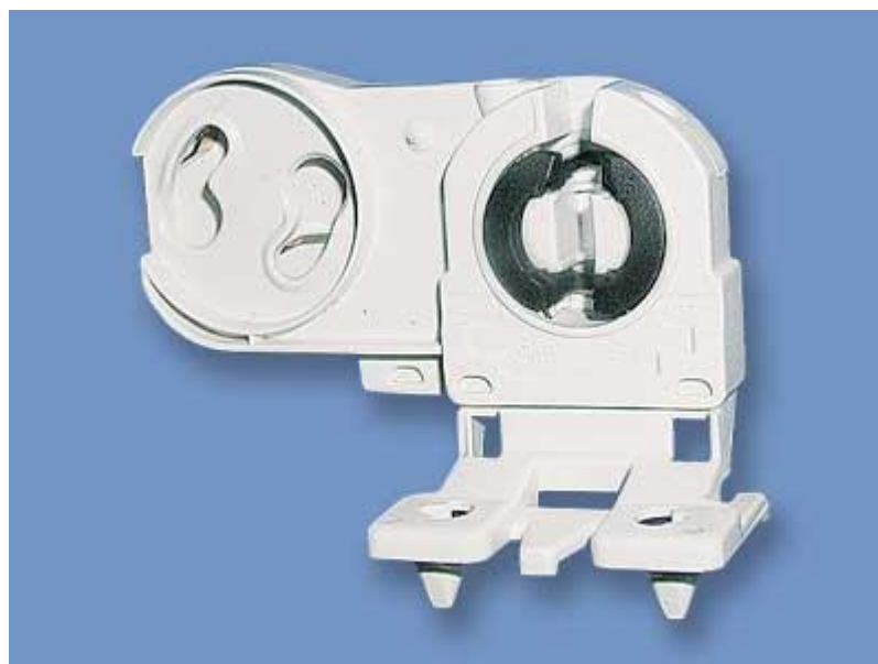
Патрон (ламподержатель) G13, вставной с лицевой стороны, h-оси 24mm, для T8 люминесцентных ламп, со стартеродержателем (крепление на цапфы)
