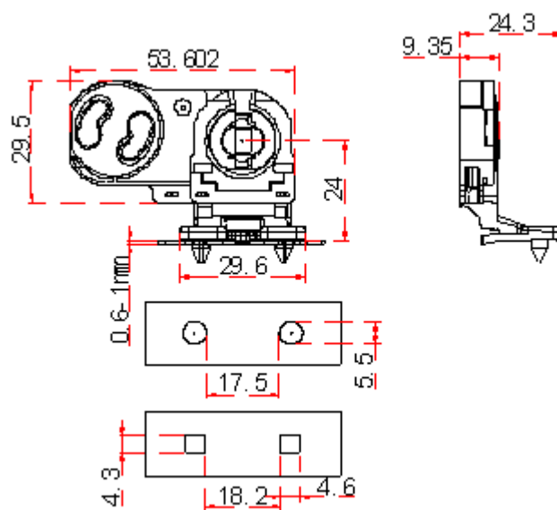
Патрон (ламподержатель) G13, вставной с лицевой стороны, h-оси 24mm, для T8 люминесцентных ламп, со стартеродержателем (крепление на цапфы)
