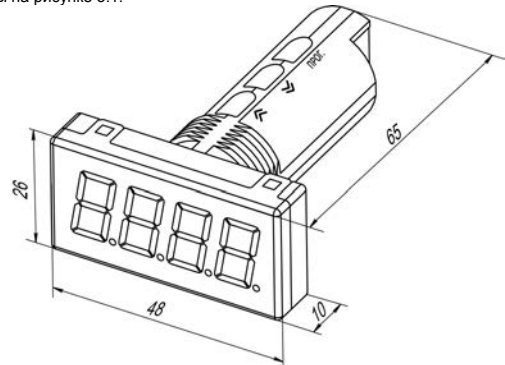
Рисунок 3.1 – Габаритный чертеж корпуса прибора
