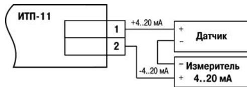
Рисунок 8.2 - Схема подключения активного датчика к ИТП-11 и другому измерителю одновременно
