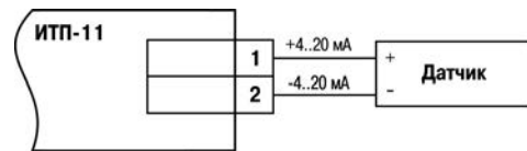
Рисунок 8.1 - Схема подключения датчика к ИТП-11
